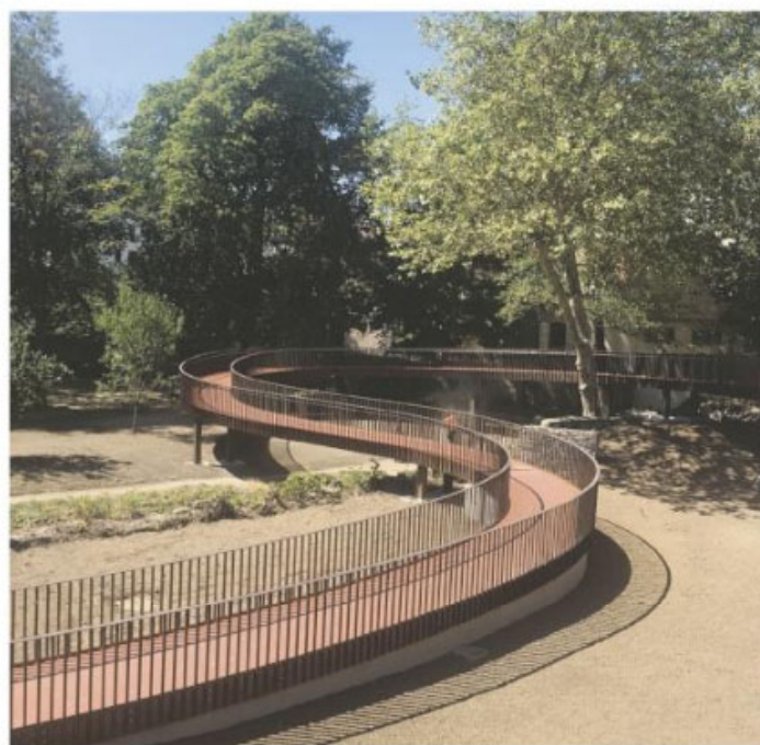
Construite en acier Corten, d'une longueur de 100 m, la passerelle de l'Arquebuse est accessible aux personnes à mobilité réduite.
